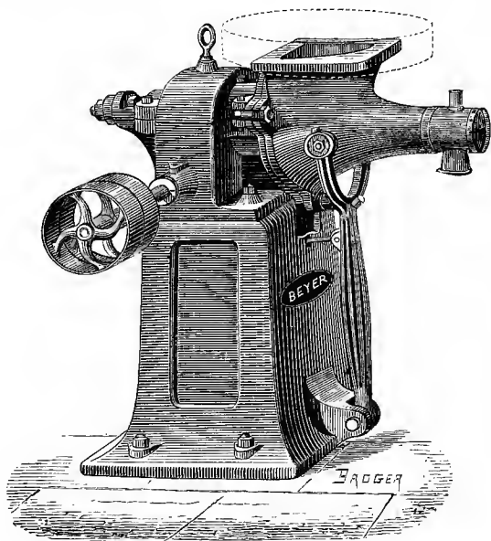
ROLLING-MACHINE ( modeleuse ).
